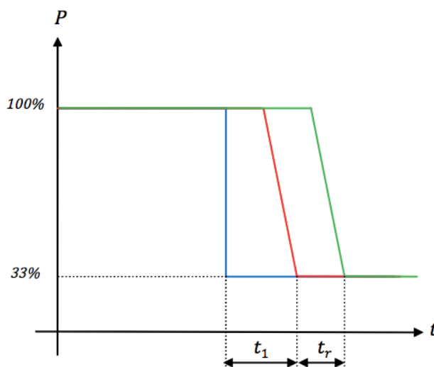
Figura 5: Exemple de temps de resposta del sistema davant una desconexió de càrrega del 100% al 33% amb un o dos generadors (blau-potència consumida per la càrrega, vermell-potència produïda en una instal·lació amb un generador, verd-potència produïda en instal·lacions amb dos generadors)
