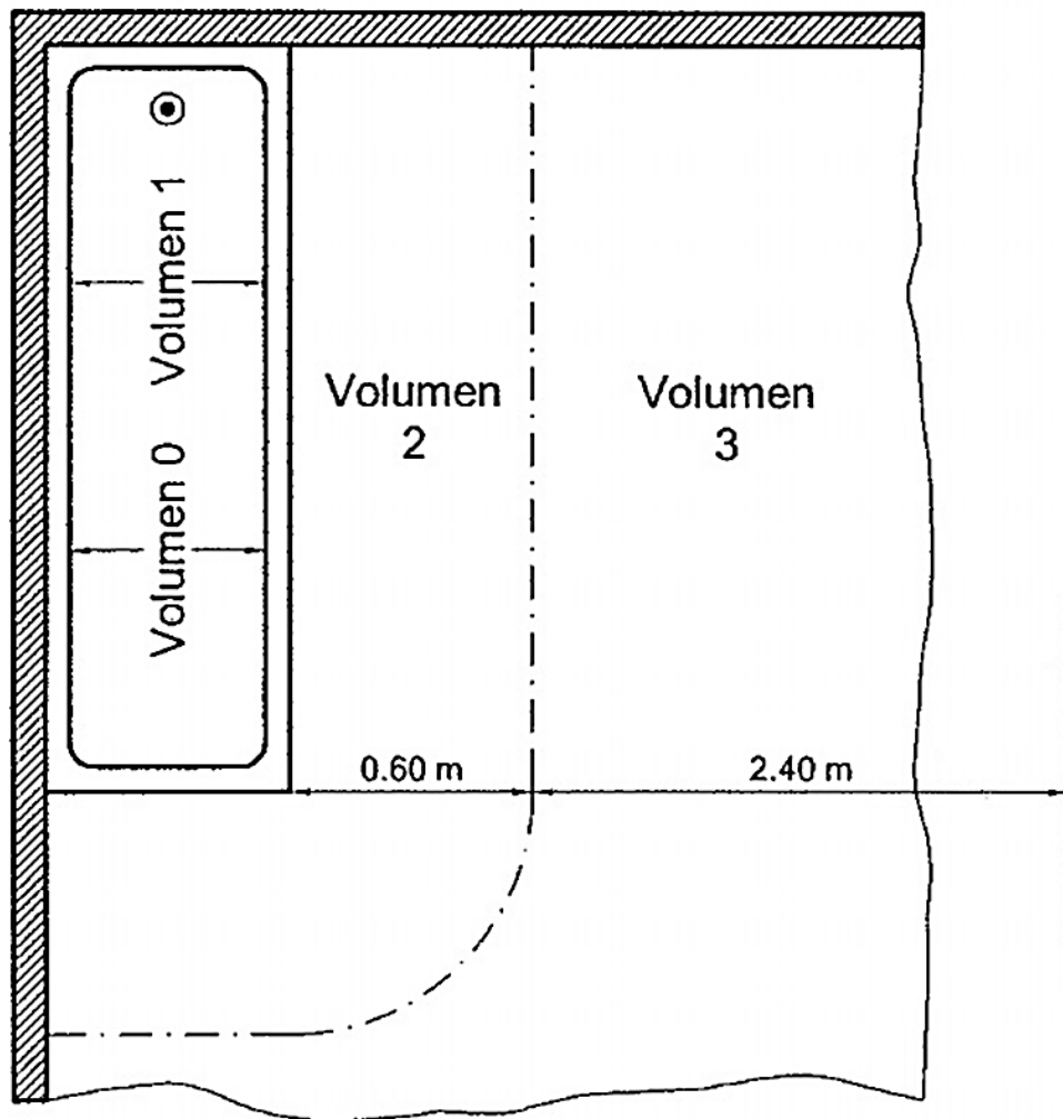
Figura 1. BAÑERA
