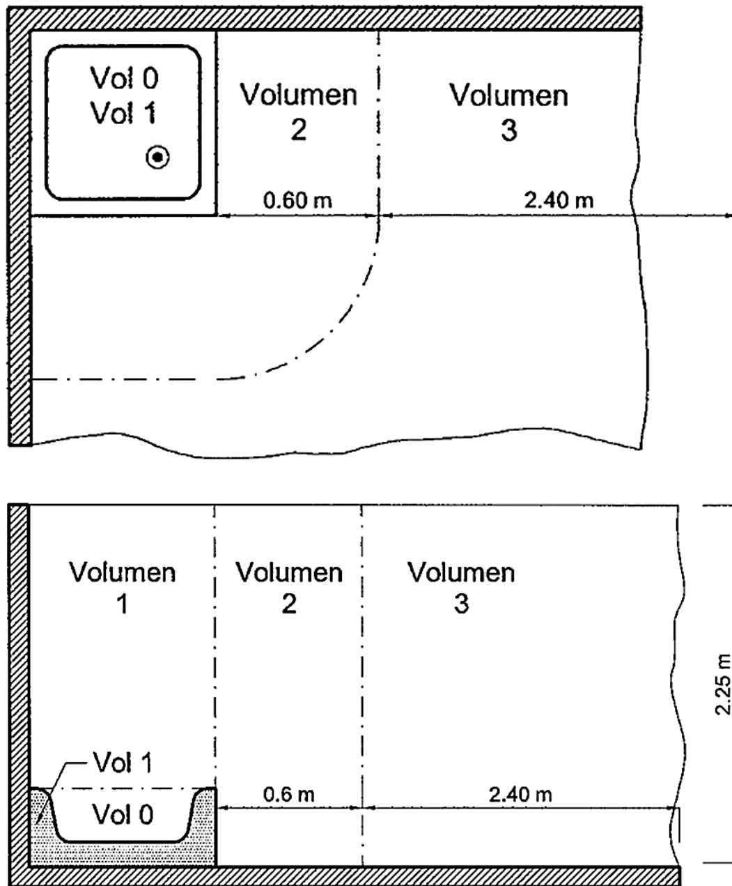
Figura 3. DUCHA
