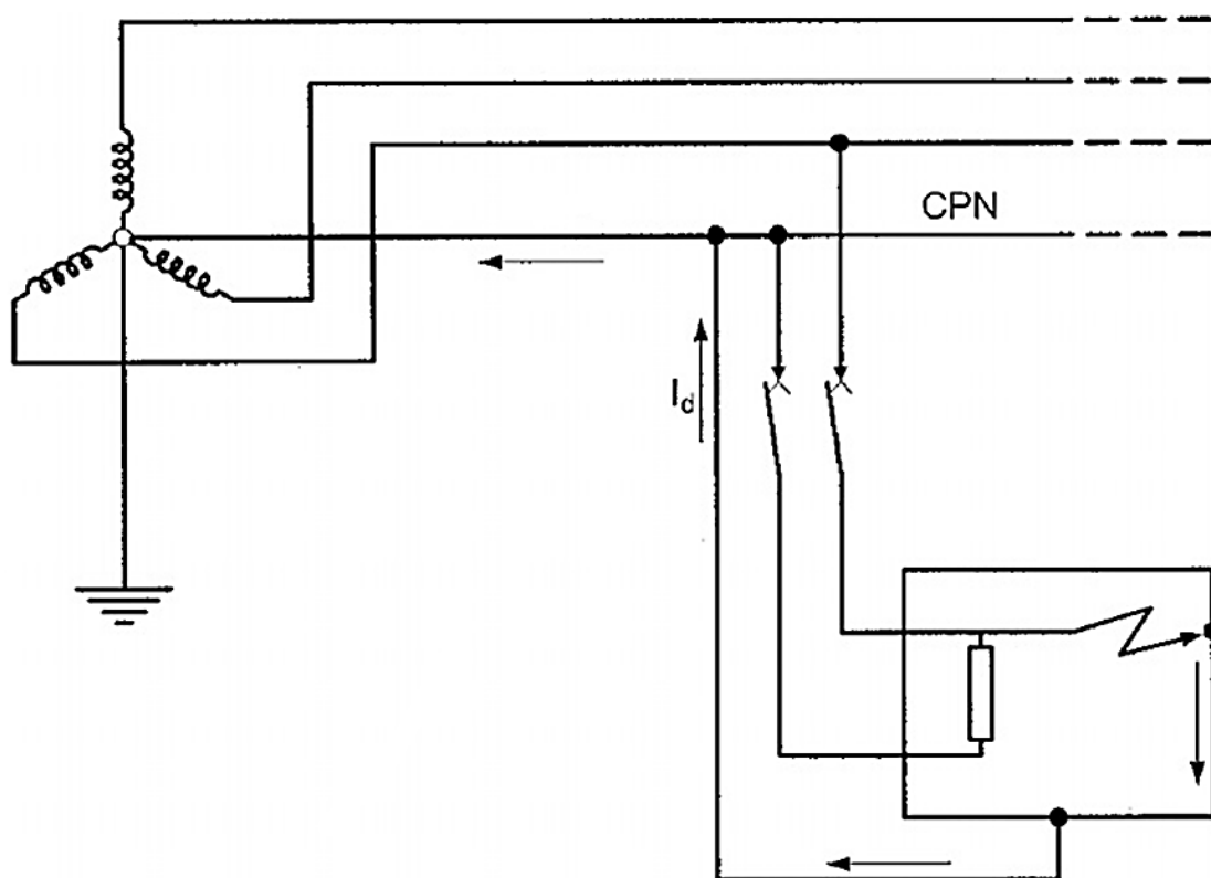
Figura 2. Esquema TN-C
