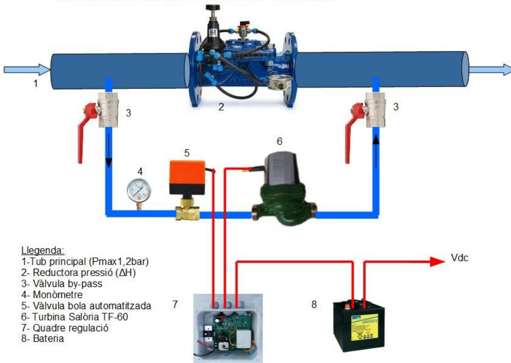
TURBINA SALORIA TF-60 AMB BY-PASS
