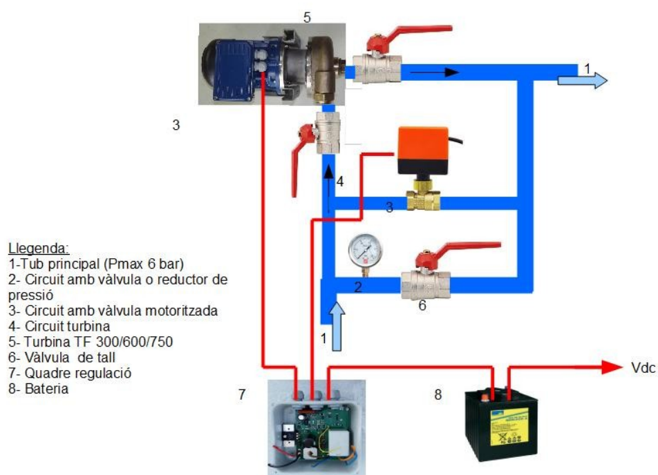
TURBINA SALÒRIA TF-300/600/750 AMB DOBLE BY-PASS
