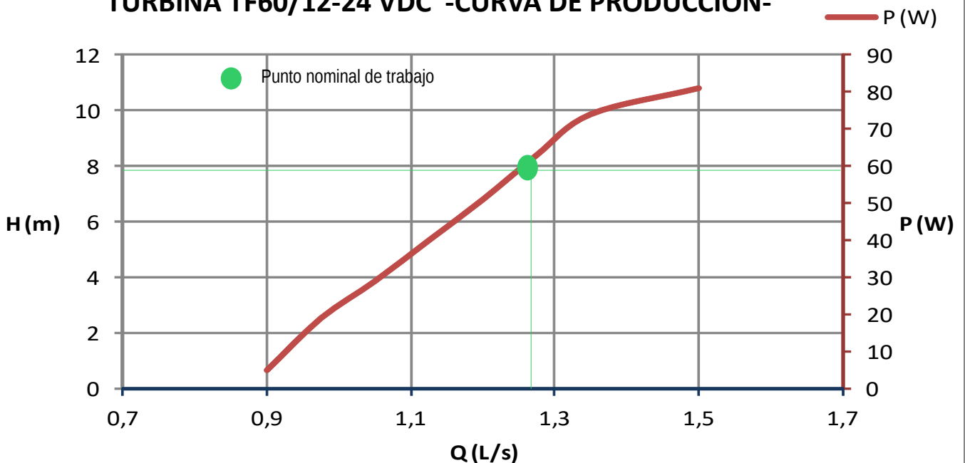
TURBINA TF60/12-24 VDC -CURVA DE PRODUCCIÓN-
