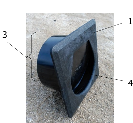
Drenolor para IMBORNAL
